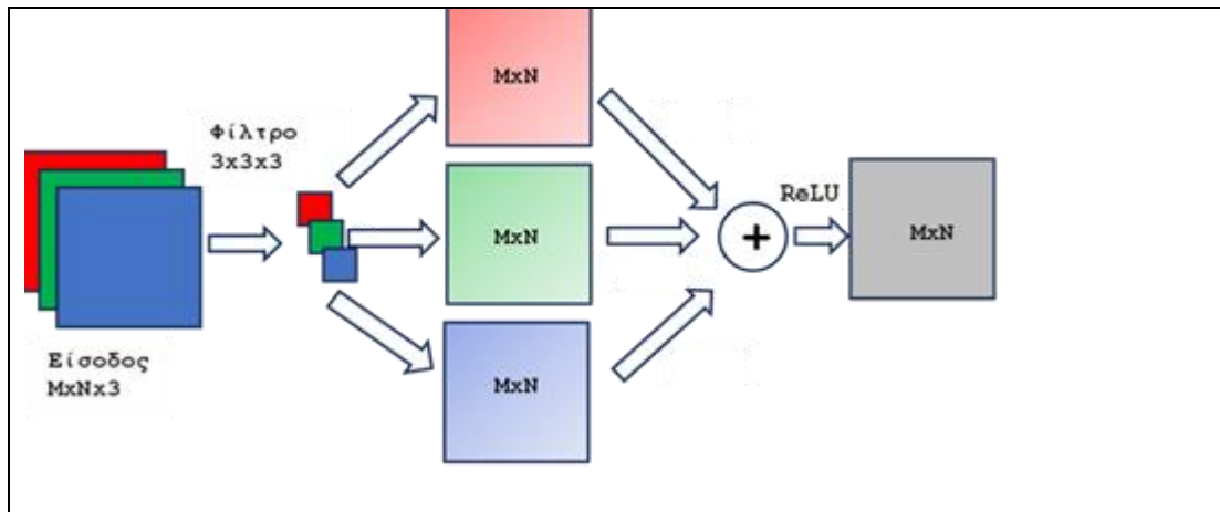
Σχ.3.4.3. Η εφαρμογή ενός φίλτρου σε είσοδο τριών καναλιών στο συνελικτικό επίπεδο
