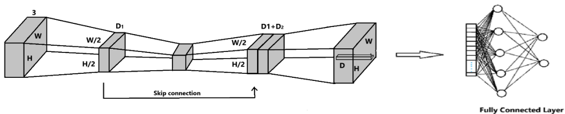
Σχήμα 3.4.1.7: Διάγραμμα των συνδέσεων (skip connections).
