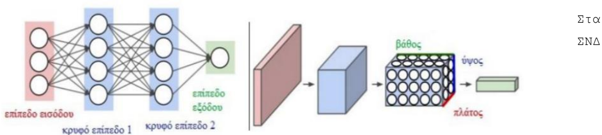
Σχήμα 3.4.1. (Αρχιτεκτονική CNN)
