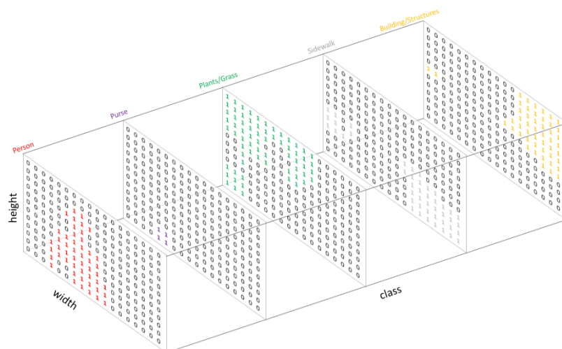
Σχήμα 3.4.1.3:Πίνακας κατάρτησης για μια εικόνα εισόδου πριν εφαρμοστεί η argmax.
