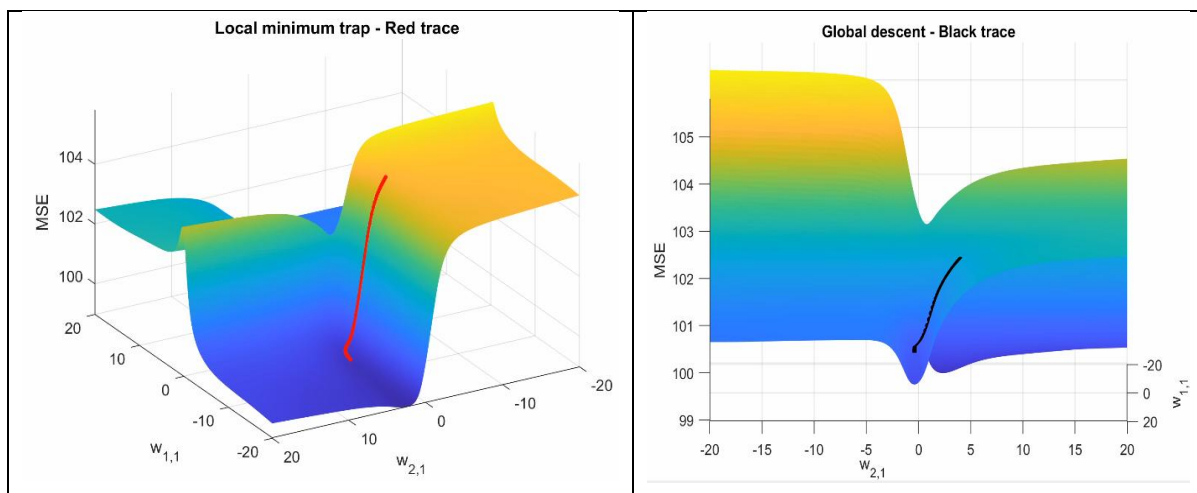
Σχήμα: Συνάρτηση κόστους.
