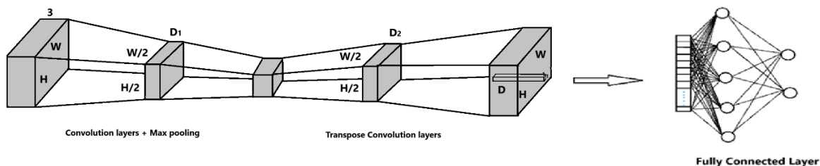
Σχήμα 3.4.1.5: Εφαρμογή επιπέδων ΑΣ έπειτα από χρήση ΣΕ
