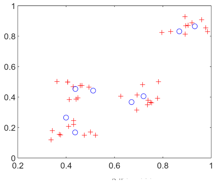
Σχήμα 4.3.3: Οκτώ νευρώνες (μπλε κύκλοι) αντιπροσωπεύουν τα δεδομένα.
