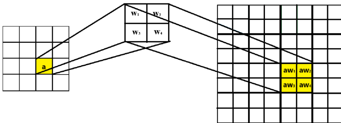
Σχήμα 3.4.1.4: Ολίσθηση του φίλτρου σε έναν πίνακα A με βήμα 2.
