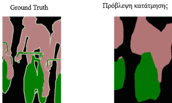
Σχήμα 3.4.1.6: Πρόβλεψη σημασιολογικής κατάτμησης ενός πλήρους συνελικτικού δικτύου.
