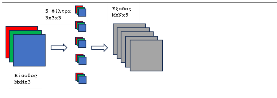
Σχ.3.4.4. Συνελικτικό επίπεδο με πέντε (5) φίλτρα
